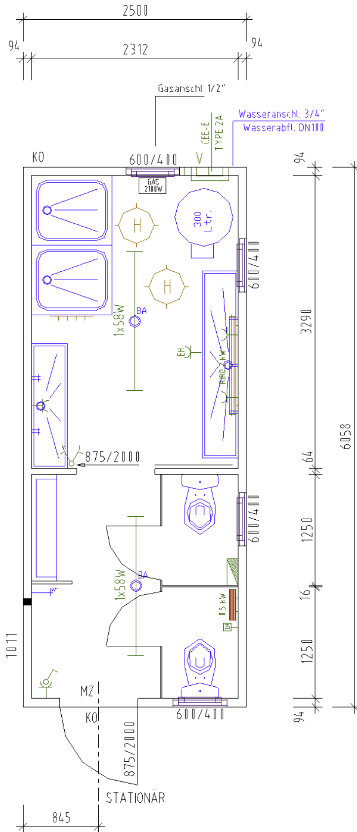
TYP SBL 6-7R Container Sanitär
