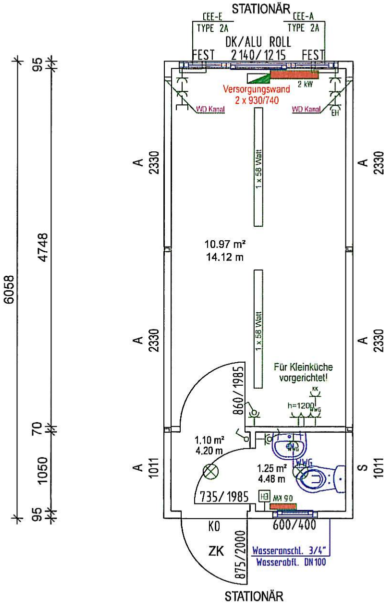
TYP SBL A6-1.2 Container Leer mit WC im Windfang
