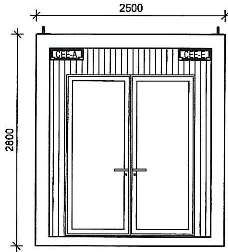
Aussenansicht SBL A WE2 Container Flur WE mit ALU-Tür
