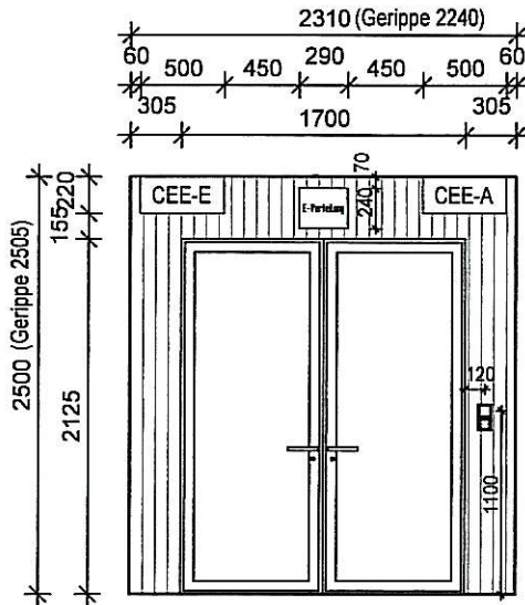
Innenansicht SBL A WE2 Container Flur WE mit ALU-Tür
